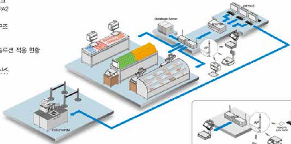
▲ 유무선 혼용 네트워크 설계
